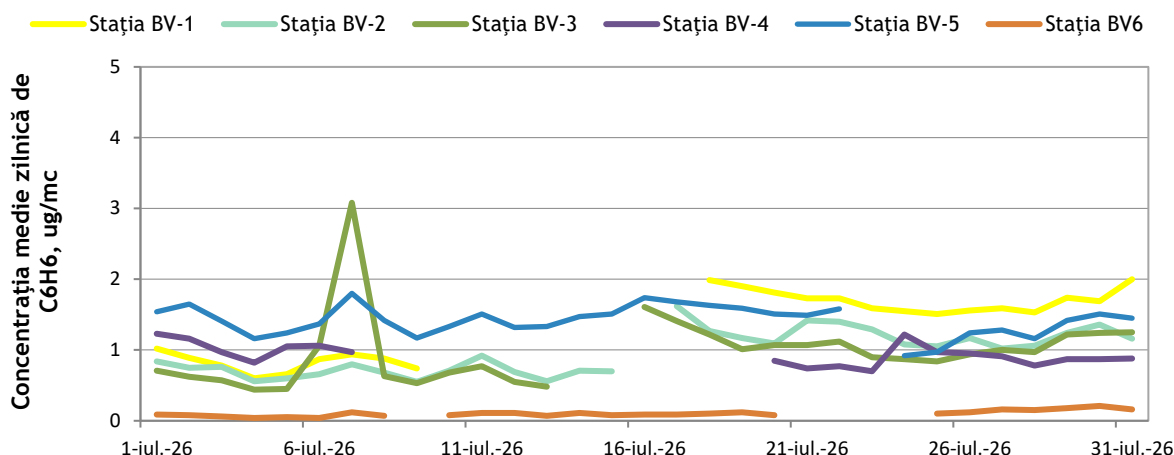
Figura 7. Evoluția concentrațiilor medii zilnice de benzen în luna iulie 2026
