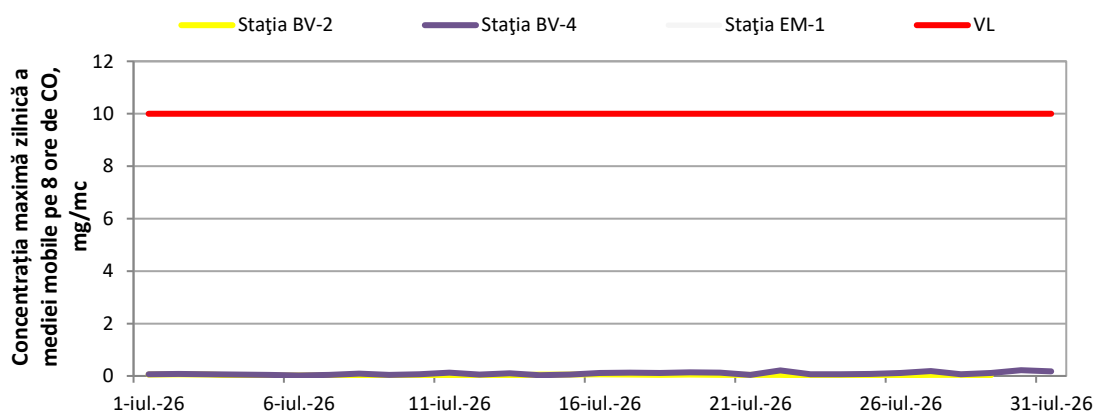
Figura 4. Concentrația maximă a mediei mobile pe 8 ore de CO în luna iulie 2026
