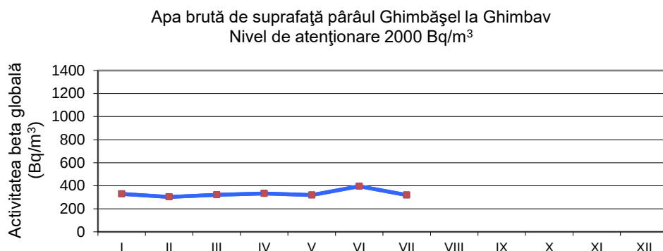
Figura 18. Activitatea beta globală imediată pentru apa de suprafață Pârâul Ghimbășel
