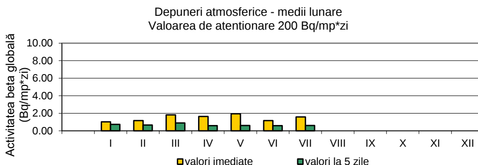
Figura 17. Activitatea beta globală pentru depuneri atmosferice
