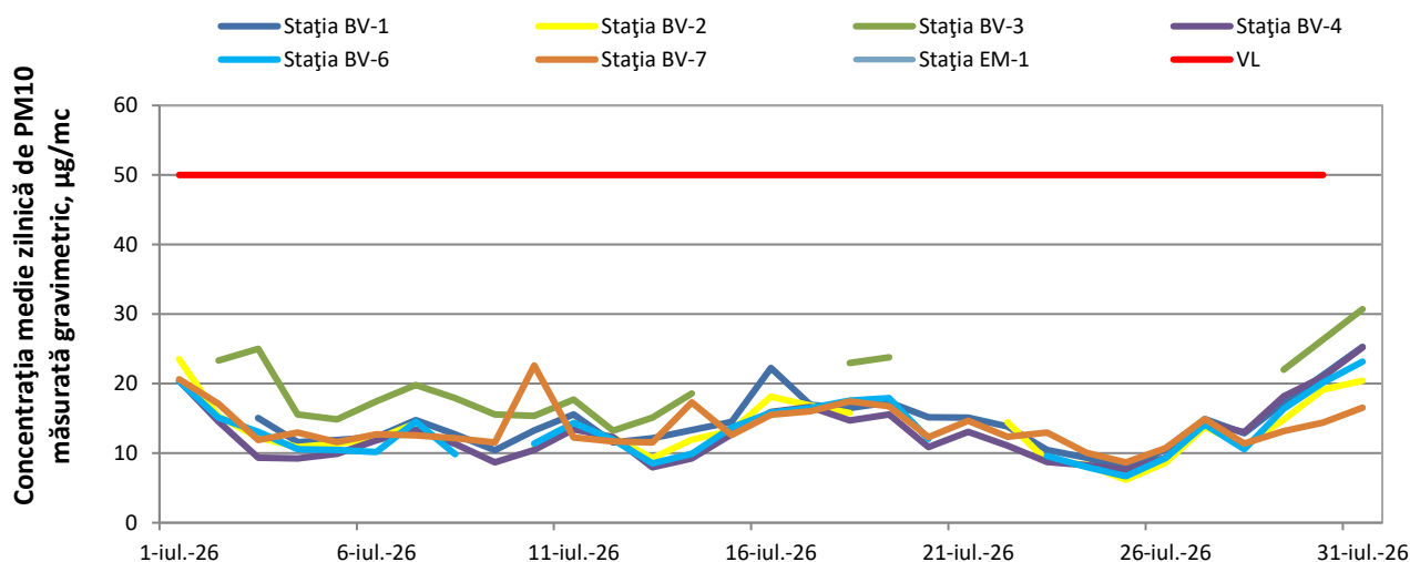
Figura 8. Evoluția concentrațiilor medii zilnice de PM10 (gravimetric) în luna iulie 2026
