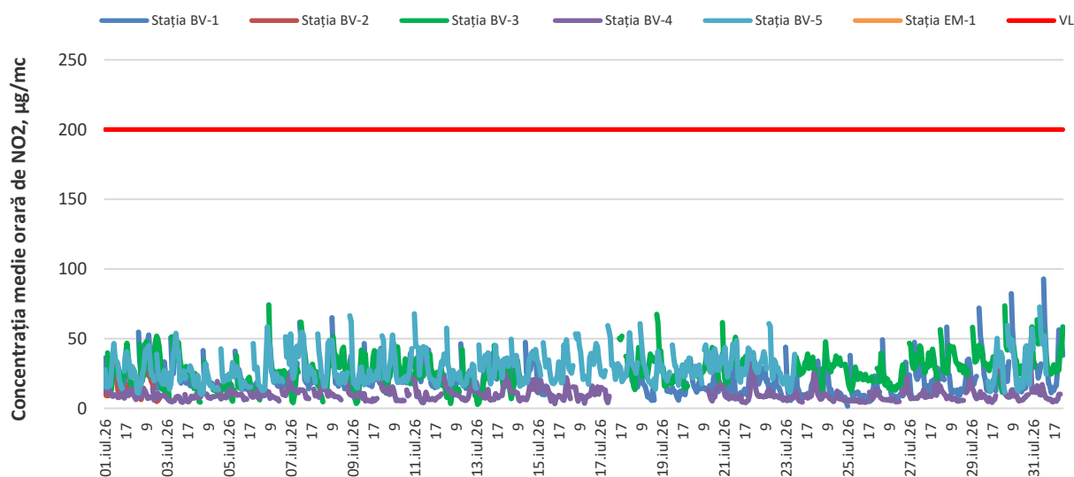
Figura 3. Concentrații medii orare de NO 2 în luna iulie 2026
